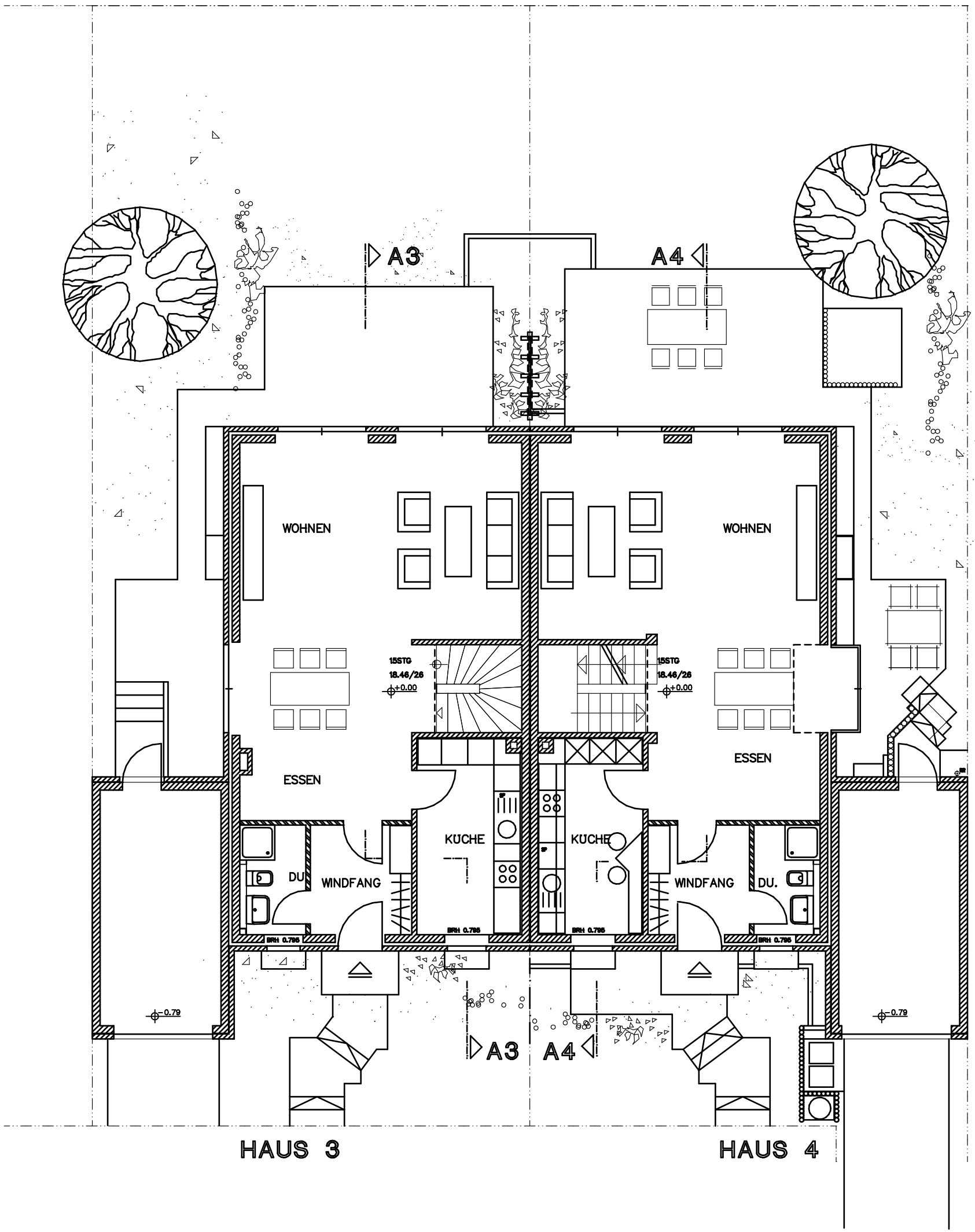
GRUNDRISS ERDGESCHOSS
