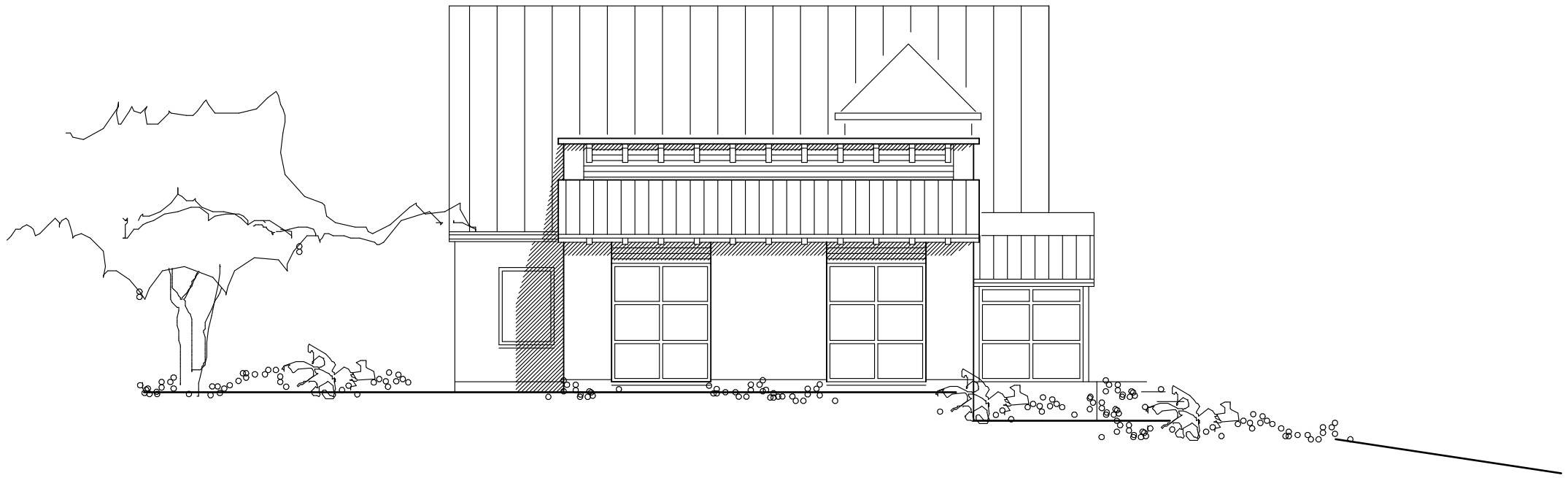
WESTANSICHT
