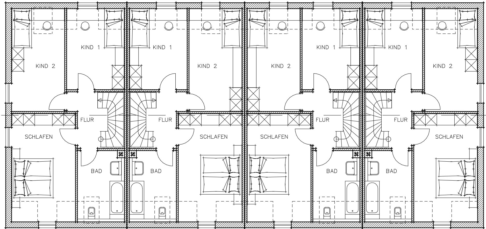
GRUNDRISS OBERGESCHOSS
