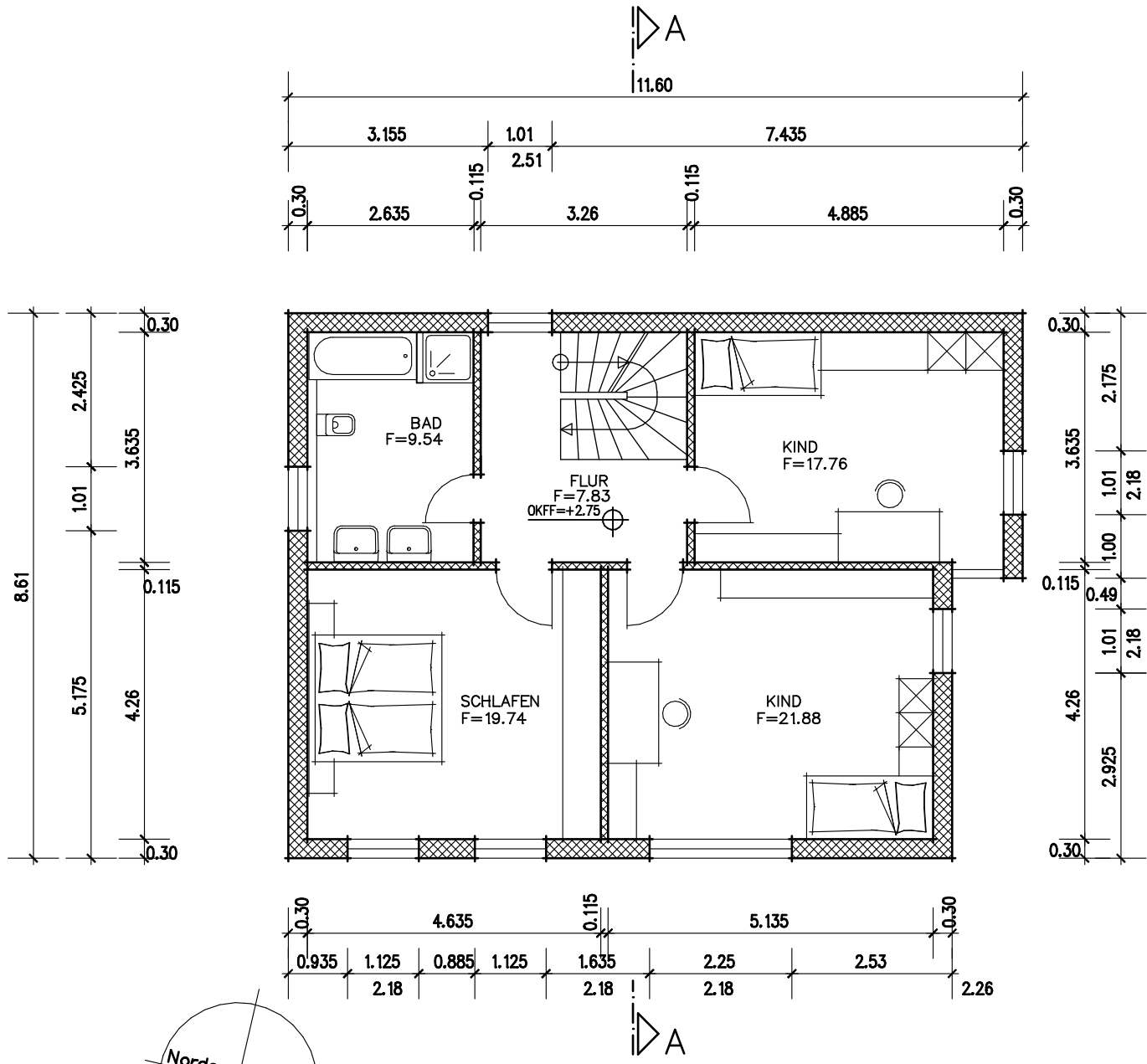
GRUNDRISS OBERGESCHOSS
